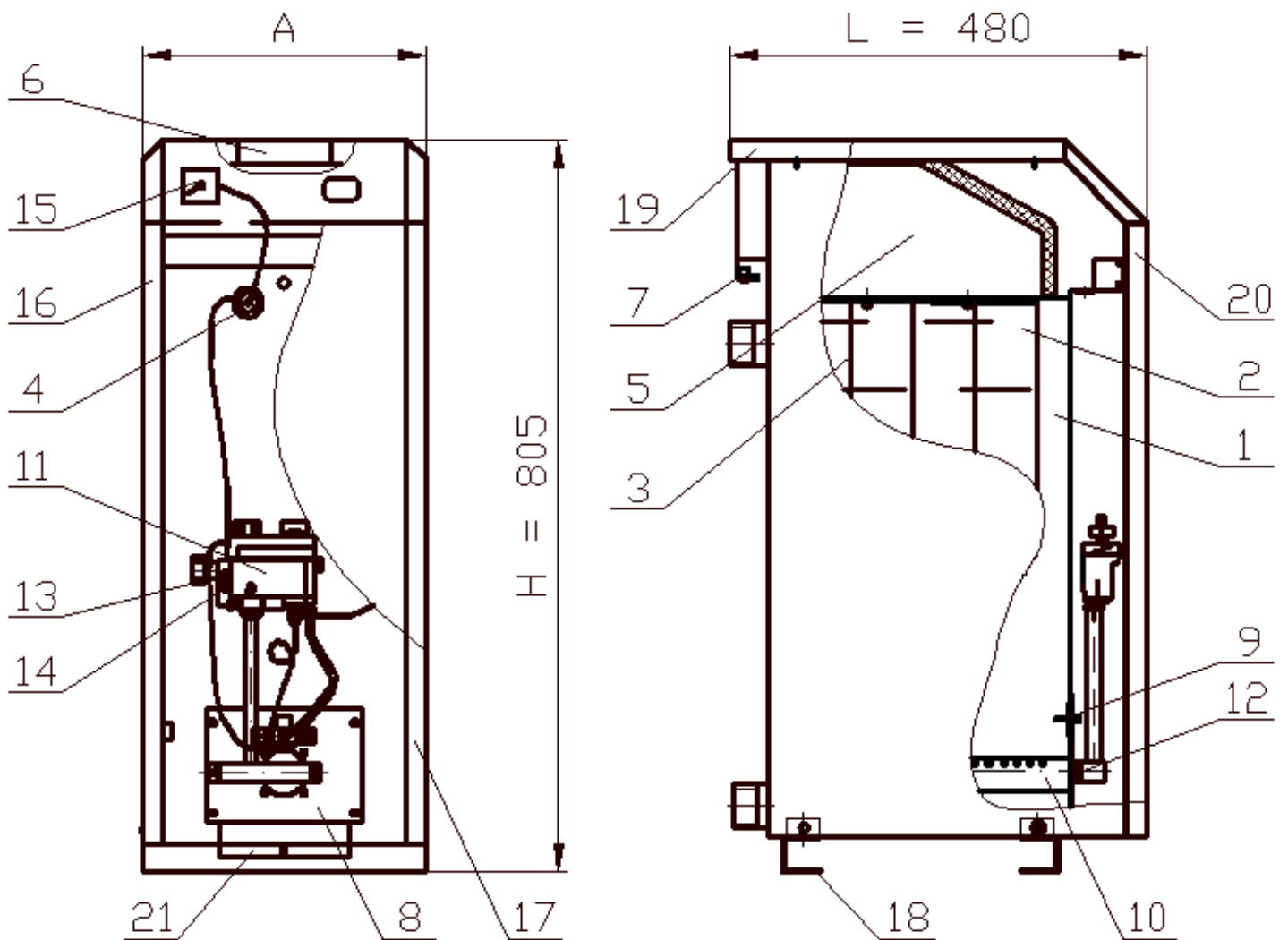
Рисунок 1. Котел опалювальний сталевий АОГВ-10КС/КСВ, АОГВ-12КС/КСВ, АОГВ-16КС/КСВ, АОГВ-20КС
