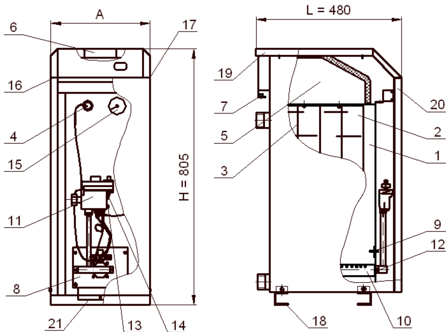
Рисунок 2. Котел опалювальний сталевий АОГВ-10КСС/КСВС, АОГВ-12КСС/КСВС, АОГВ-16КСС/КСВС, АОГВ-20КСС/КСВС
