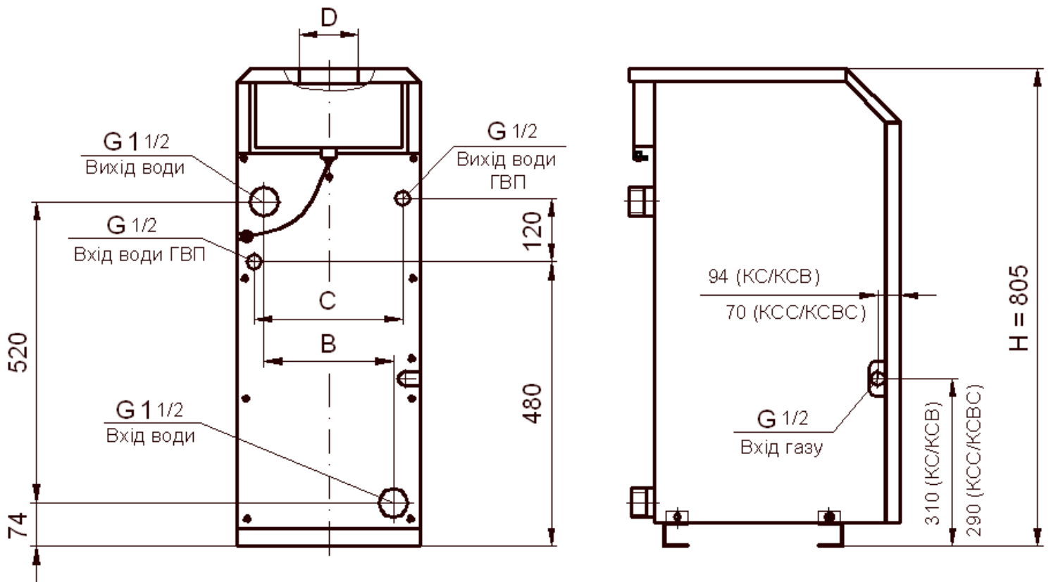
Рисунок 3. Приєднувальні розміри котлів опалювальних сталевих типу АОГВ ( вид ззаду)
