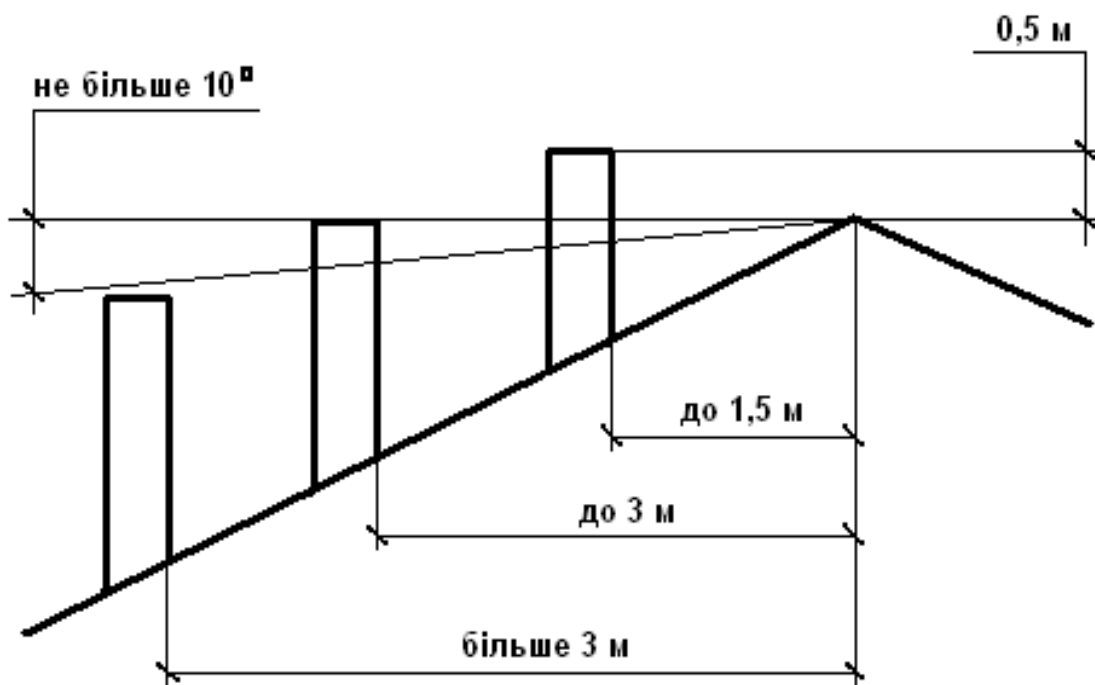
Рисунок 6. Розміщення димоходу
