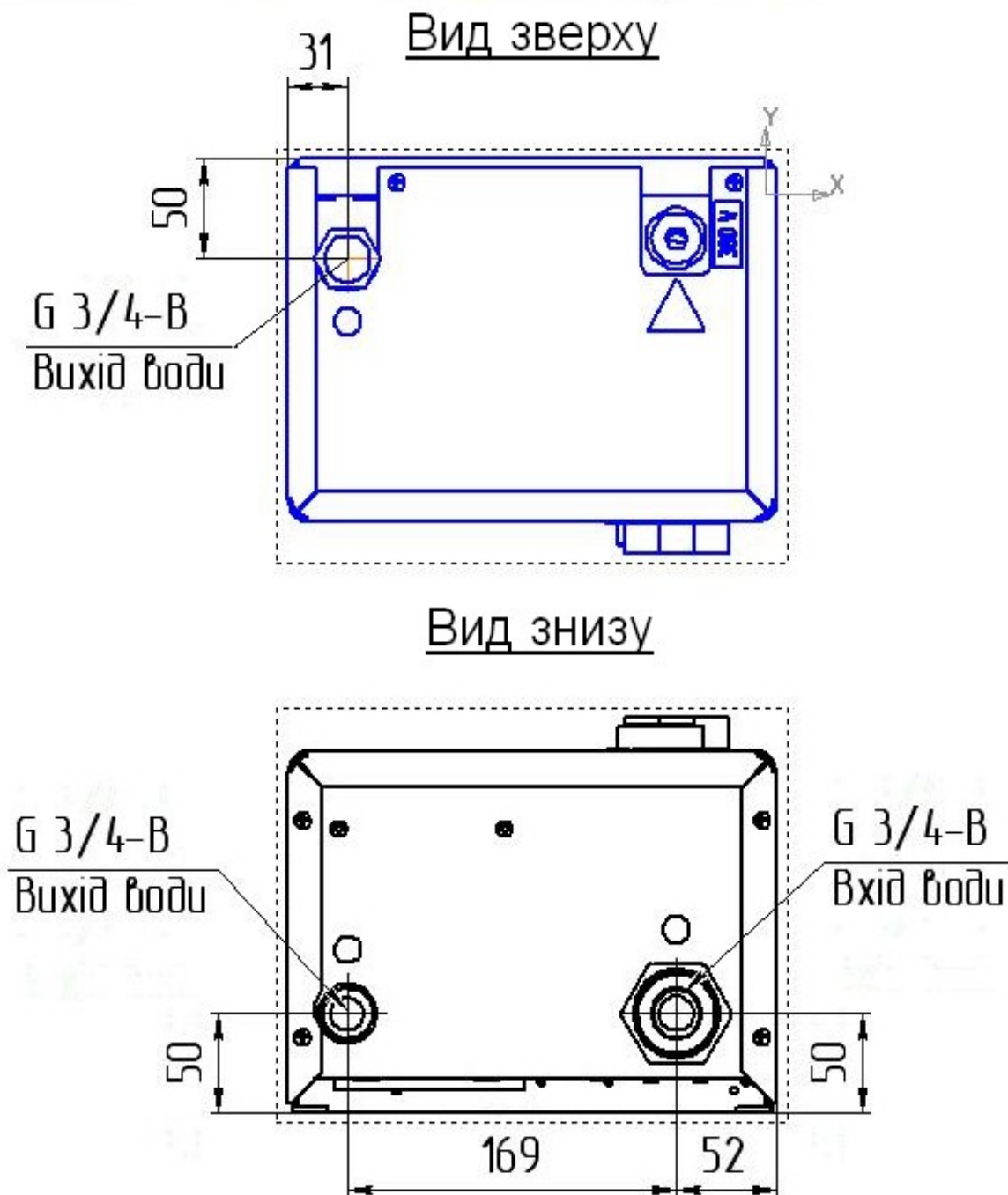
Рисунок 3. Приєднувальні розміри.
