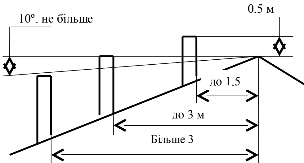
Рисунок 3. Розміщення димоходу
